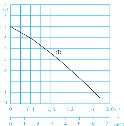
性能曲线
